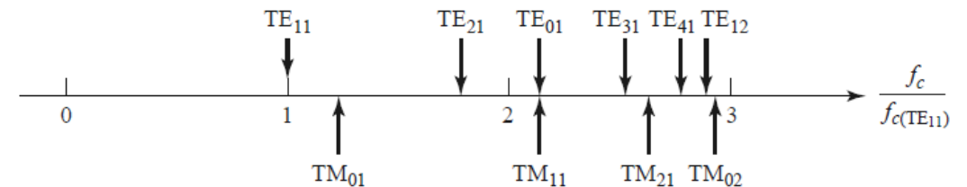
(Fig. 3.13 of Pozar)
