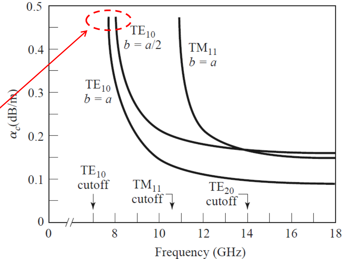
(Fig. 3.12 of Pozar)
